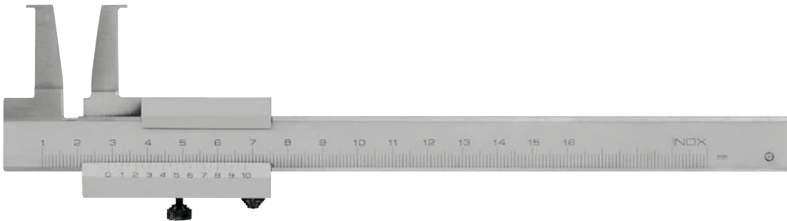
Calibro per gole interne Nonio 1/20. Lettura 0,05 mm. Corsoio con vite di bloccaggio. Scala cromata opaca.
